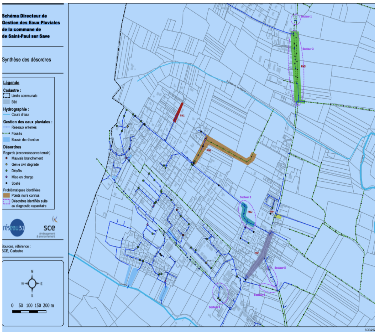
Fig. 2 Schéma Directeur de Gestion des Eaux Pluviales de la commune de Saint-Paul-sur-Save Programme d'actions des eaux pluviales urbaines
